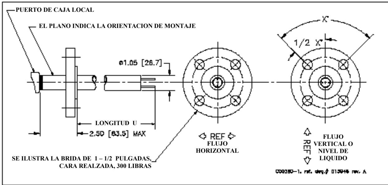
Figura A – 7. Conexión Bridada al Proceso
